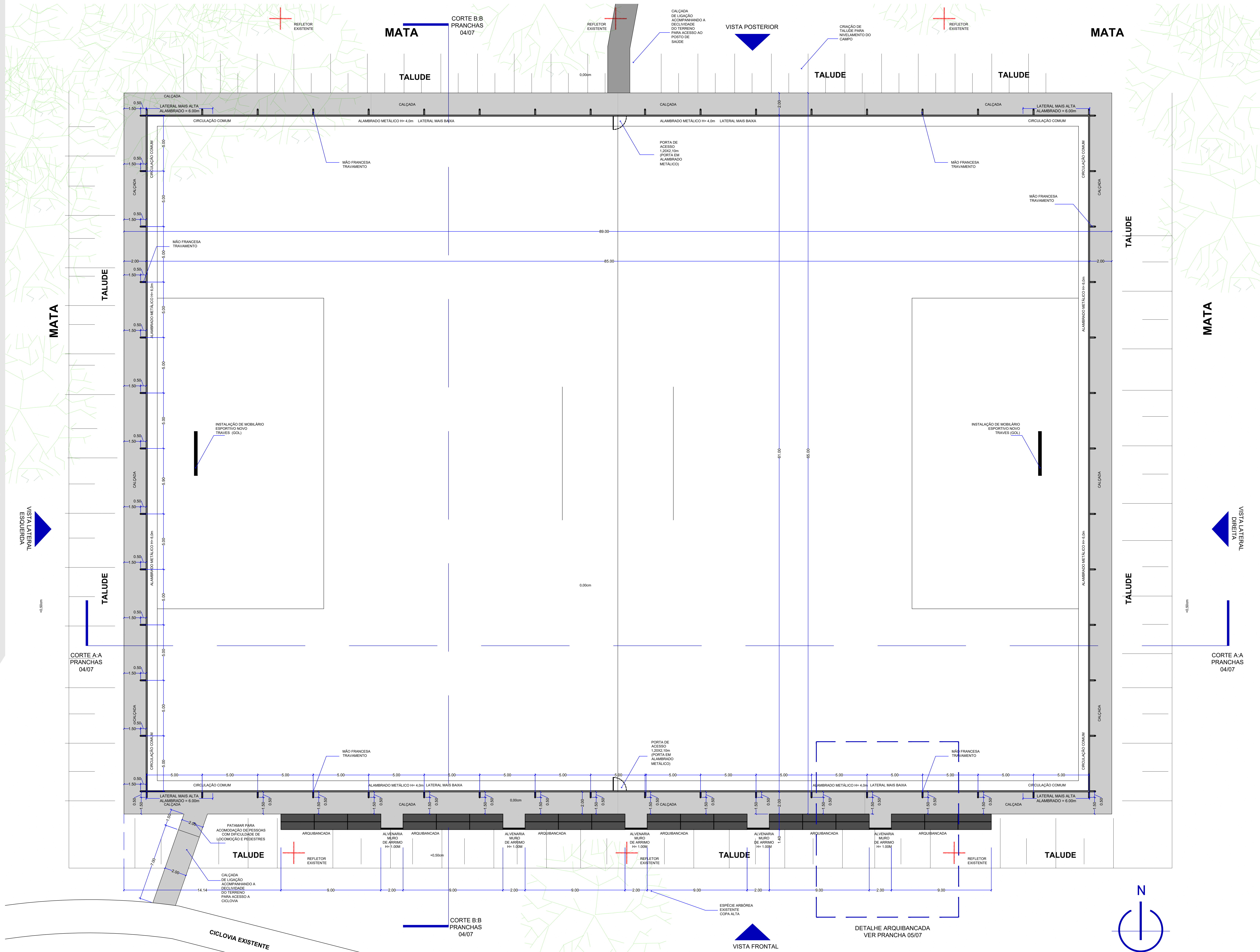
PLANTA BAIXA - CAMPO SOCIETY - PARQUE DO BOSQUE ESC.: 1/125
