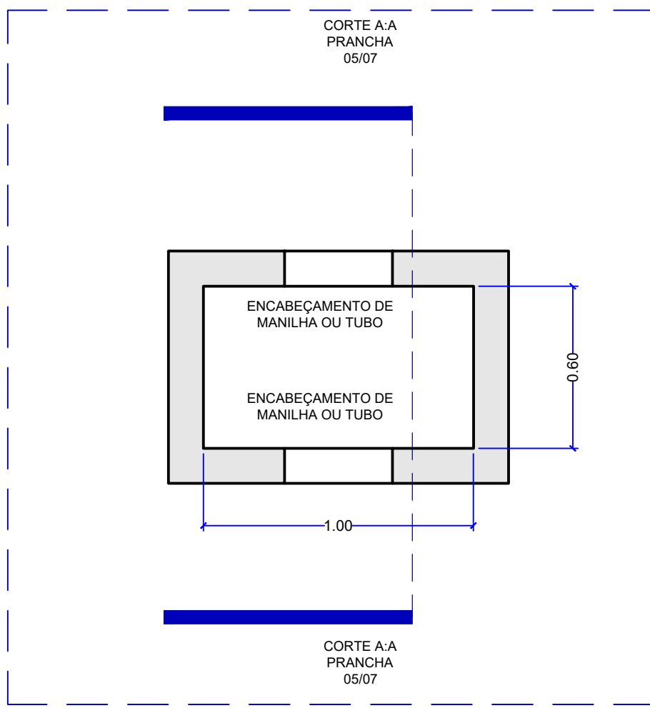
DETALHE 06 - PLANTA BAIXA - CAIXA DE INSPEÇÃO ESC.: 1/20
