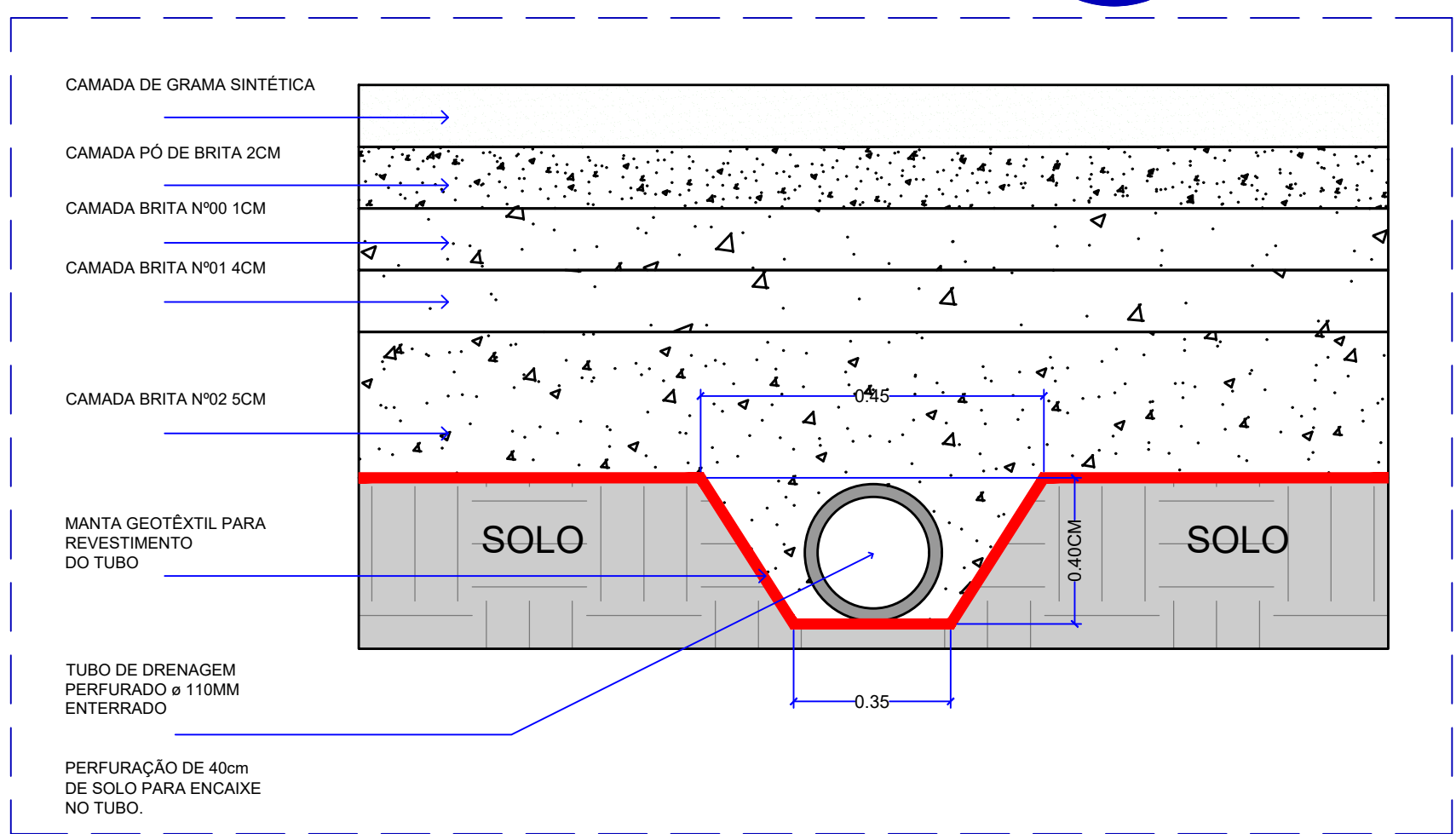
DETALHE 08 - CORTE DA BASE DRENANTE TUBO PEAD ESC.: sem escala
