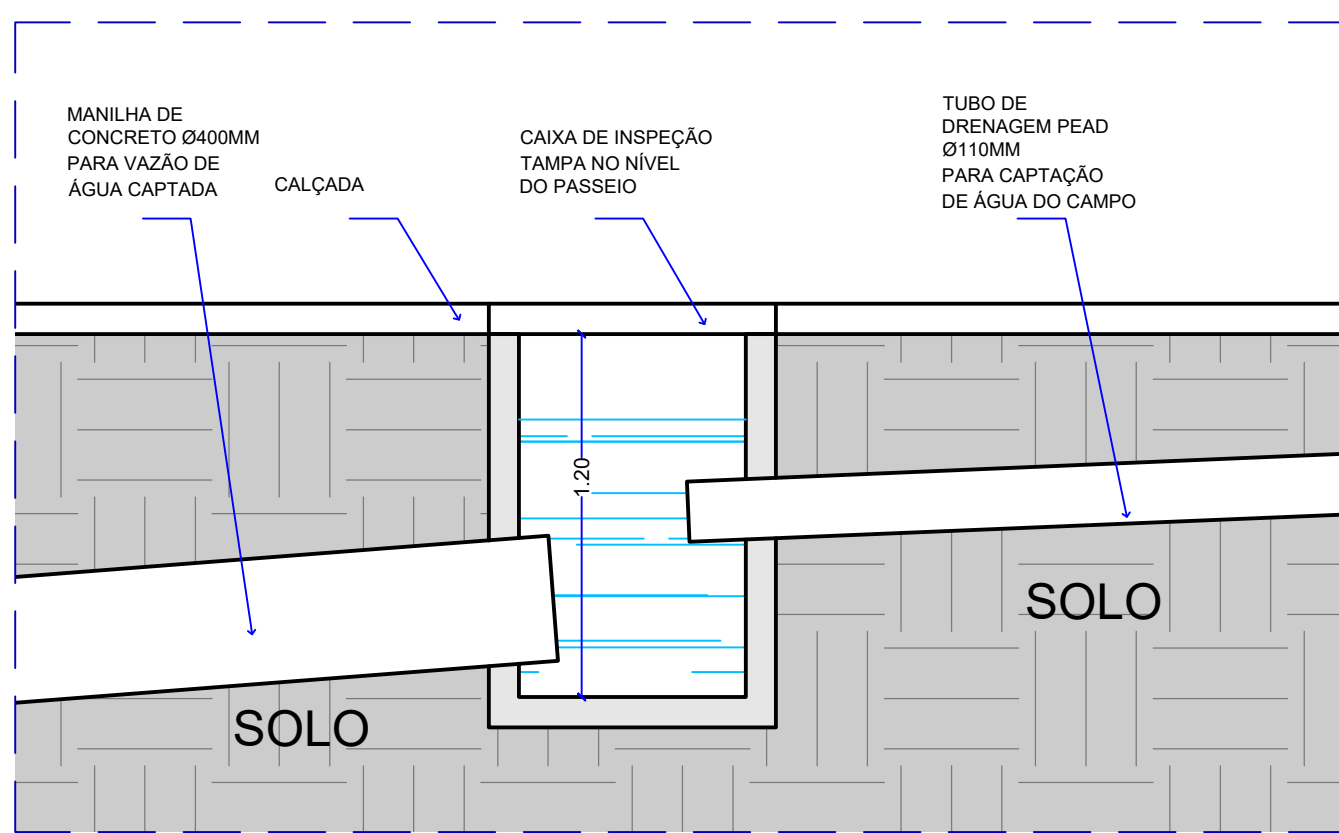
DETALHE 07 - CAIXA DE INSPEÇÃO ÁGUAS PLUVIAIS (MANILHAS DE CONCRETO) ESC.: SEM ESCALA
